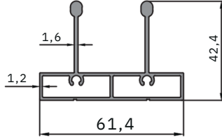
2'li Sürme Yan Kasa 2 Way Sliding Side Frame Profile Profili 0.463 kg/m
