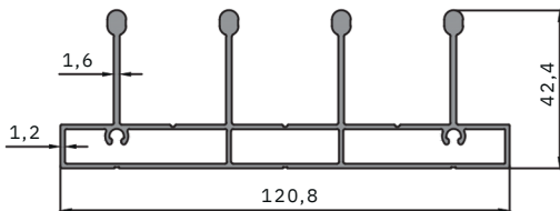
Eşikli 4'lü Sürme Alt Kasa 4 Way Sliding Bottom Frame With Threshold Profili 1.683 kg/m
