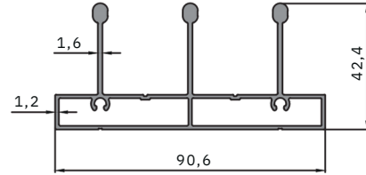
Eşikli 3'lü Sürme Alt Kasa 3 Way Sliding Bottom Frame Profile With Profili 1.287 kg/m
