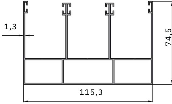
Silinebilir Isıcam Baza Wipeable Insulating Heat Glazing Plinth Profili 0.490 kg/m
