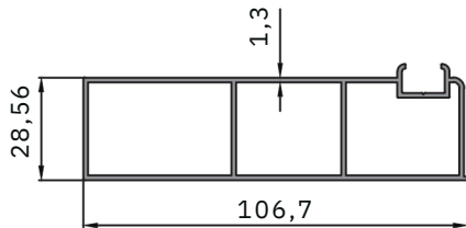
Silinebilir Alt Kasa Profili Erasable Bottom Frame Profile 1.168 kg/m
